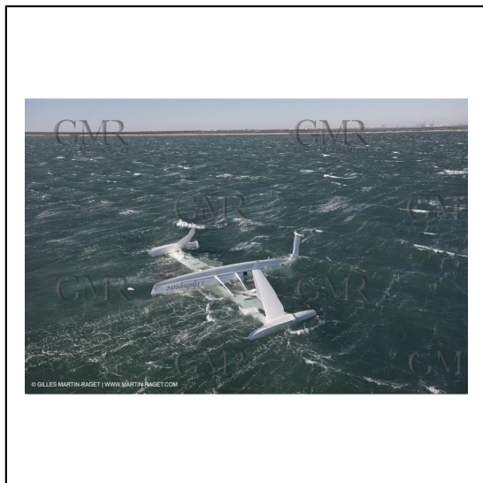
21/12/2008 - Port Saint Louis du Rhône (FRA, 13) - L'Hydroptère peu après son chavirage survenu lors d'une tentative contre le record de vitesse absolu à la voile*** 21/12/2008 - Port Saint Louis du Rhône (South of France) - The Hydroptere just after its capsize when trying to beat the overall sailing speed record
