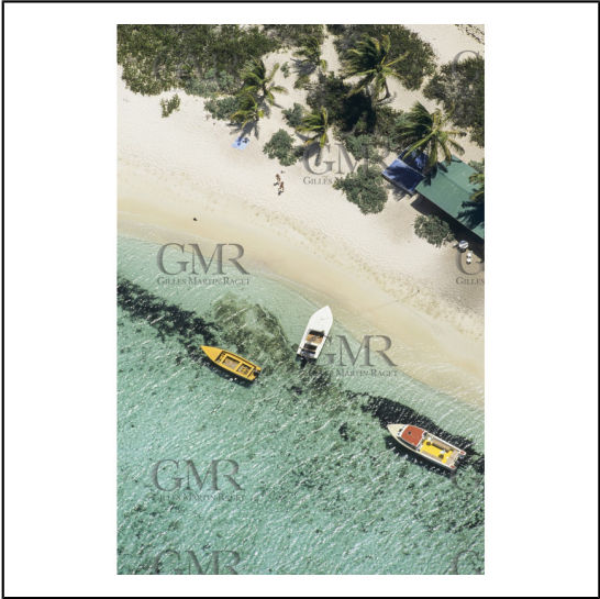
ScanJan151689.JPG
