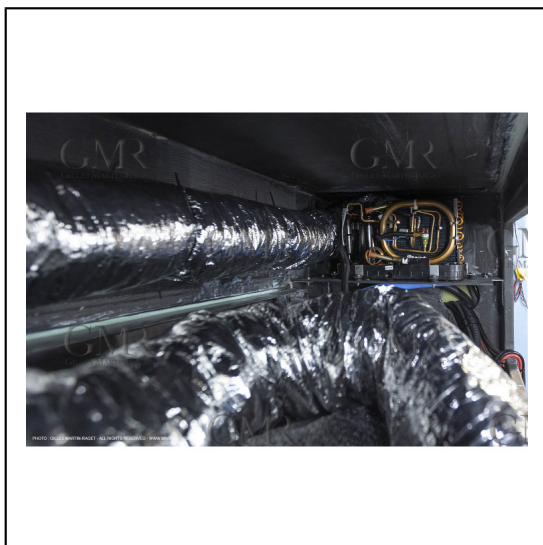
29/10/2018, La Grande Motte (FRA,30), Chantier Gunboat, construction du Gunboat 68, système air conditionné
