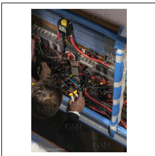
29/10/2018, La Grande Motte (FRA,30), Chantier Gunboat, construction du Gunboat 68, montage panneaux électriques
