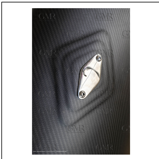
29/10/2018, La Grande Motte (FRA,30), Chantier Gunboat, construction du Gunboat 68, détail tube mât
