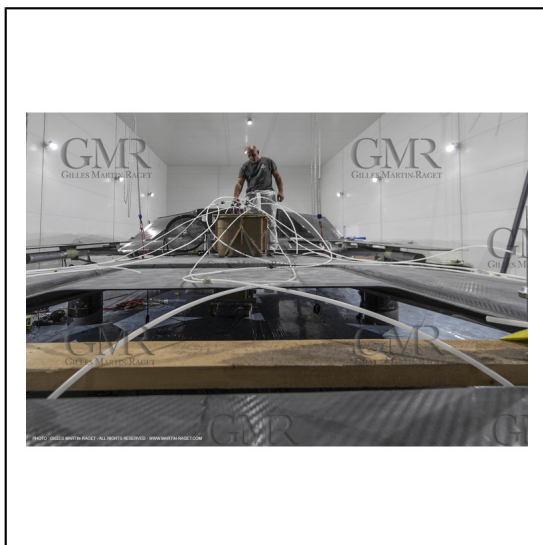
29/10/2018, La Grande Motte (FRA,30), Chantier Gunboat, construction du Gunboat 68, préparation de l'infusion
